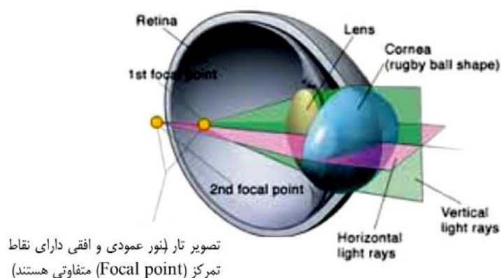
شکل ۳ تصویر مسیرهای نور در چشم آستیگماتیسم، نور در دو صفحه متفاوت (اینجا عمود بر هم) در دو نقطه متفاوت فوکس شده است.
